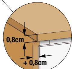
Holz-Abdeckplatte: Höhe 0,8cm
