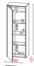
Li = Drehtür mit Linksanschlag
