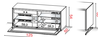
Mit Fuß H. 63 Optional (siehe Seite 28)
