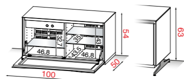
Mit Fuß H. 63 Optional (siehe Seite 28)
