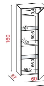
Re = Drehtür mit Rechtsanschlag
