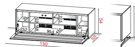
Mit Fuß H. 63 Optional (siehe Seite 28)
