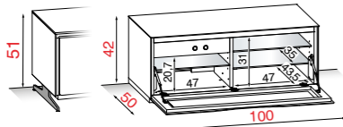
Mit Fuß H. 51 Optional (siehe Seite 28)
