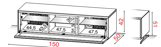
Mit Fuß H. 51 Optional (siehe Seite 170)
