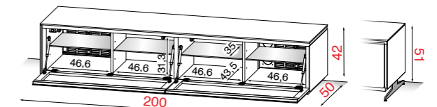
Mit Fuß H. 51 Optional (siehe Seite 170)
