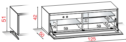
Mit Fuß H. 51 Optional (siehe Seite 28)
