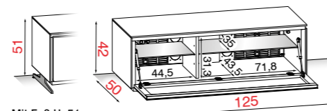
Mit Fuß H. 51 Optional (siehe Seite 170)
