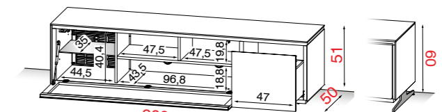
Mit Fuß H. 60 Optional (siehe Seite 170)
