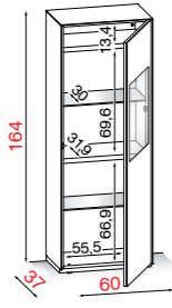
Re = Drehtür mit Rechtsanschlag
