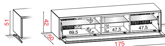
Mit Fuß H. 51 Optional (siehe Seite 170)
