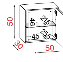
Re = Drehtür mit Rechtsanschlag
