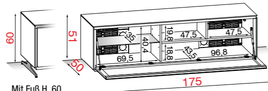
Mit Fuß H. 60 Optional (siehe Seite 170)
